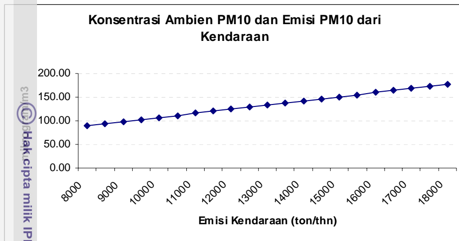
Gambar 23 Hubungan antara Konsentrasi Ambient PM_{10} dan Emisi Kendaraan
